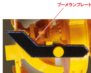
硬質地盤には基本的にブームランプレートを装着する
